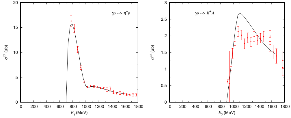
FIG. 2: \sigma^{tot} of \gamma p \rightarrow \eta p, K^+ \Lambda
