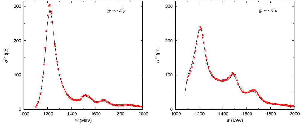
FIG. 1: \sigma^{tot} of \gamma p \rightarrow \pi^0 p, \pi^+ n
