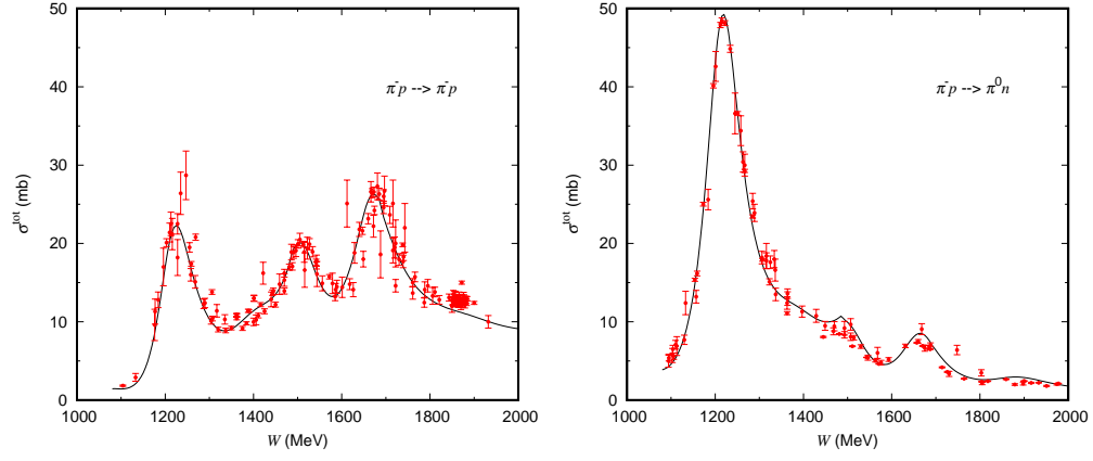
FIG. 1: \sigma^{tot} of \pi^- p \rightarrow \pi^- p, \pi^0 n
